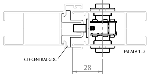
FECHAMENTO CENTRAL
