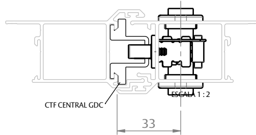
FECHAMENTO CENTRAL
