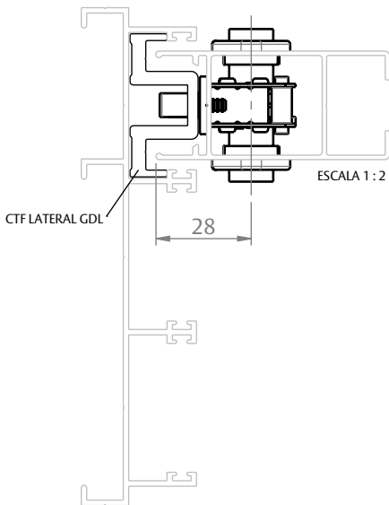
FECHAMENTO LATERAL
