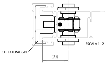
FECHAMENTO LATERAL
