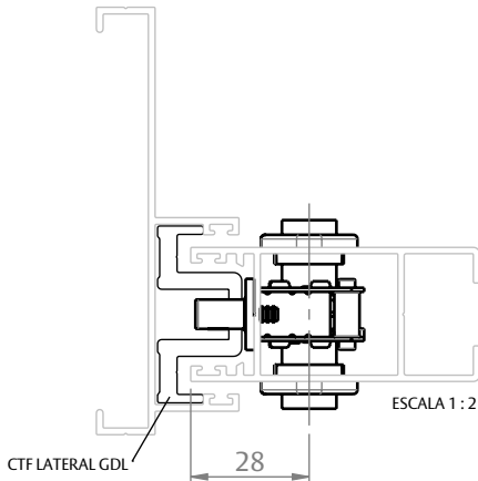
FECHAMENTO LATERAL
