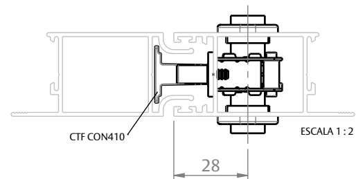
FECHAMENTO CENTRAL
